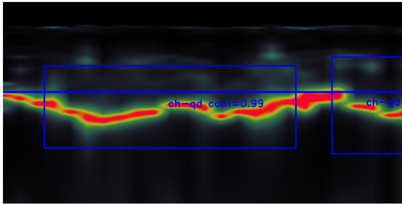
自动标识超厚或强度不足 (蓝框), 置信度 99%
