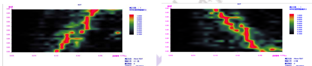
N1 测线往返 (D17 激振)
