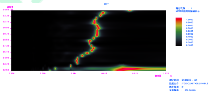
脱空云图（脱空位置已钻孔验证，深层脱空）
