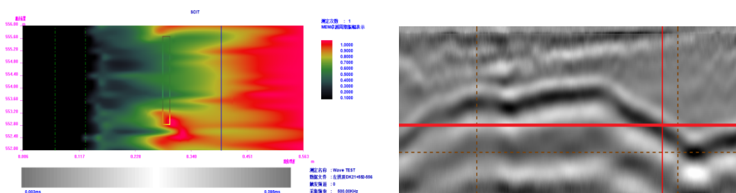
左拱腰测试图 (左: 声频 右: 雷达)
