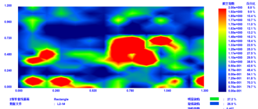
左：L2-1#测区-S31 结果图
