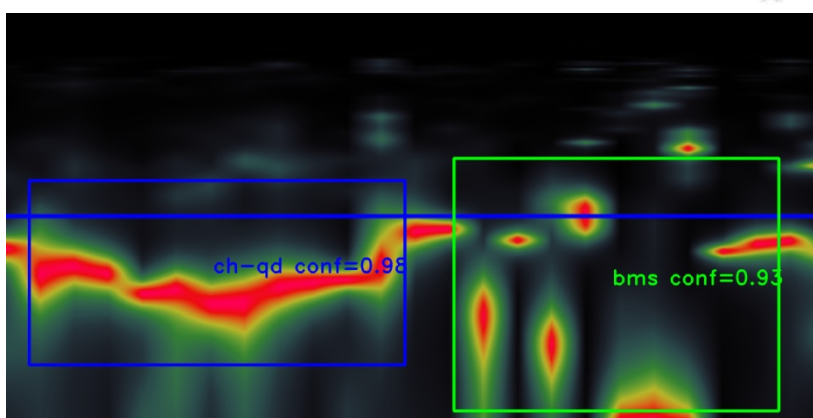
自动标识超厚/强度不足和不密实，置信度 93~98%
