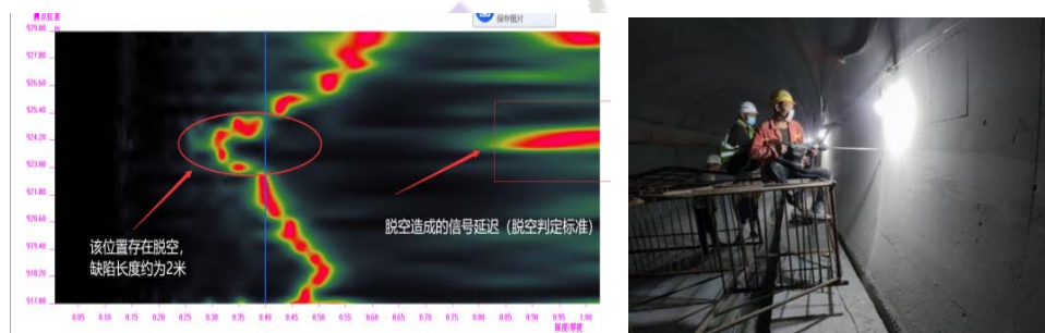
边墙测试结果图与现场钻孔验证（脱空）
