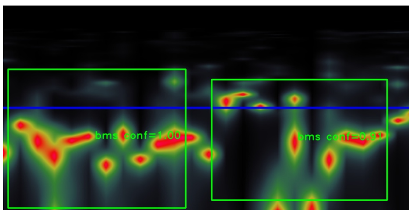
自动标识不密实（绿框），置信度 91~100%
