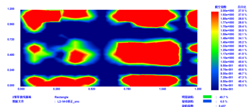
右：L2-1#测区-声频装置结果图
