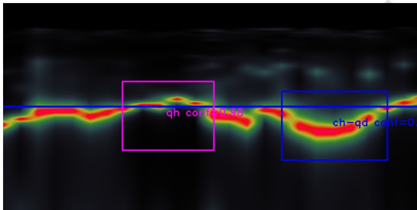
自动标识欠厚 (紫框), 置信度 96~98%
