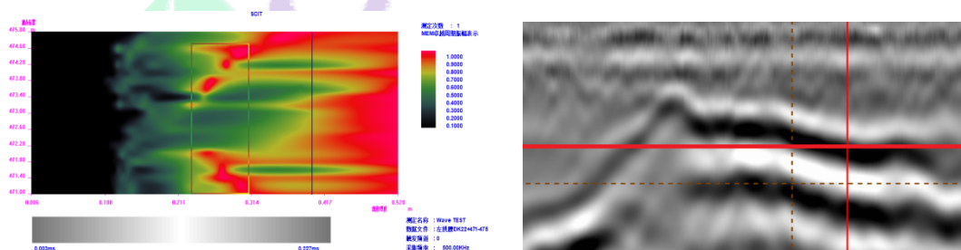
左拱腰测试图 (左: 声频 右: 雷达)
