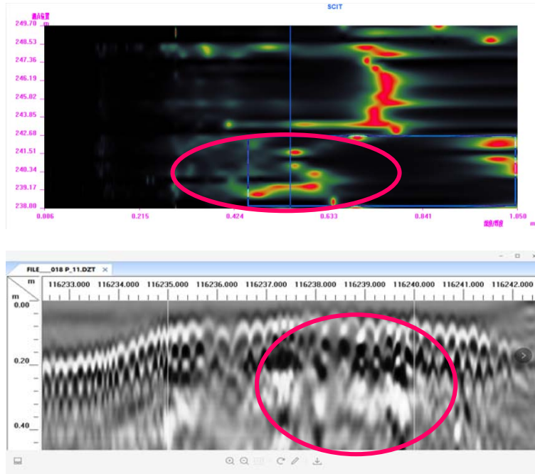
检测结果图（上：IAE、下：雷达法）
