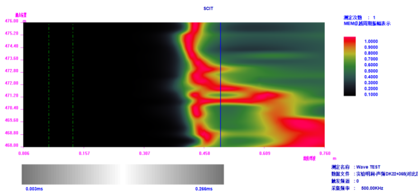
声频小车不同敲击距离 (0. 1m-0. 15m-0. 2m-0. 25m) 测试结果
